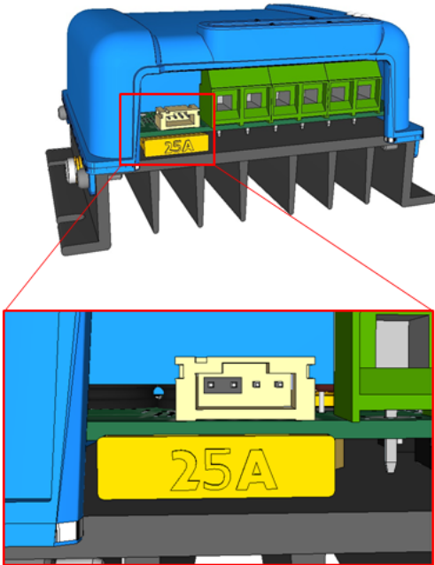
Kuva 1 b: VE.Direct-tietoliikenneportin konfigurointipinnit - 100 V mallit
