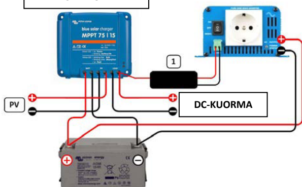
Kuva 6: Victron-inverterrimallit Phoenix 12/180, 24/180, 12/350, 24/350, Phoenix Inverter C -mallit ja MultiPlus C -mallien liitäntä edellyttää liitäntäkaapelin (1) käyttöä: "Inverting remote on-off cable" (tuotenumero ASS030550100)
