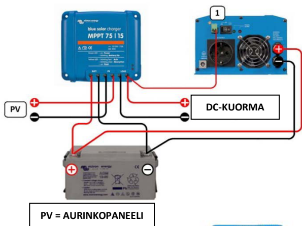
Kuva 5: Victron-inverterrimallit Phoenix 12/800, 24/800, 12/1200 ja 24/1200 ovat hallittavissa liittämällä inverterin kauko-ohjaimen oikeanpuoleinen liitin (1) suoraan aurinkopaneelilaturin kuormalähtöön. Vastaavasti, kaikki Phoenix VE.Direct-inverterit ovat hallittavissa liittämällä kauko-ohjaimen vasemmanpuoleinen
